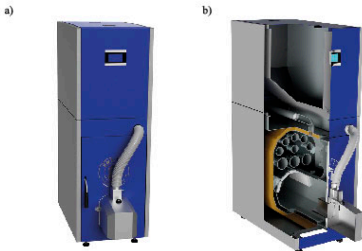
Rys. 1. Kocioł BIO COMPACT BLUE, gdzie: a) widok ogólny, b) przekrój przez kocioł
