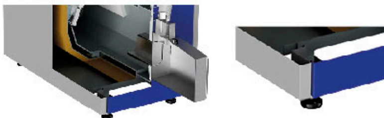
Rys. 2. Stopka regulacyjna, służąca do wypoziomowania kotła typu BIO COMPACT BLUE
