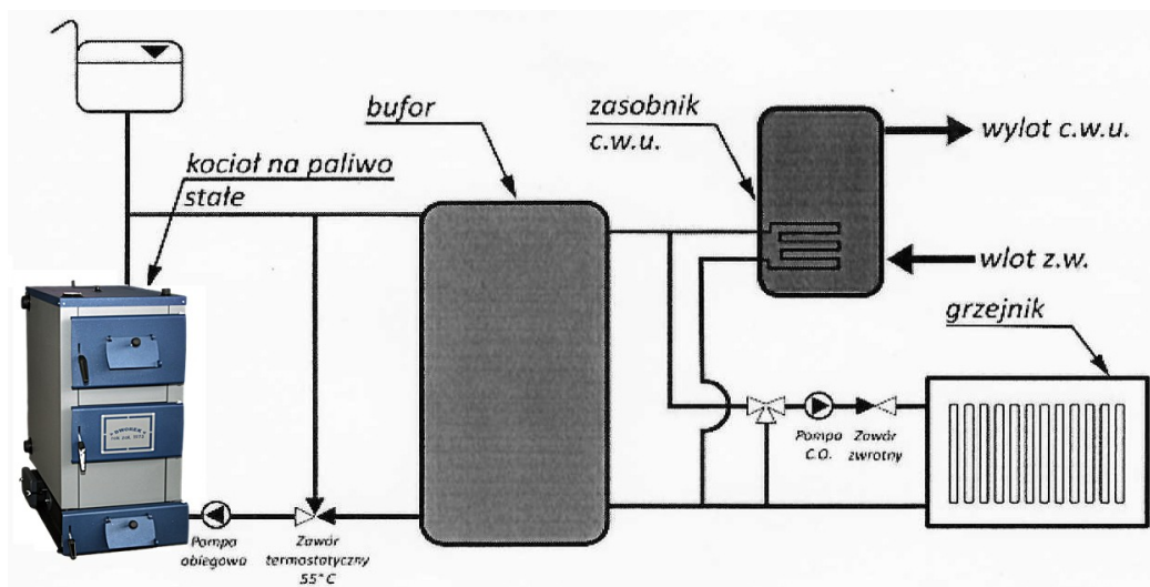
Rysunek przedstawia przykładowy schemat podłączenia kotła do instalacji grzewczej (centralnego ogrzewania) z buforem.
